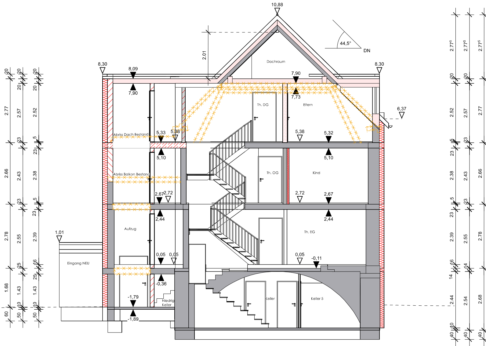
Schitt A-A
